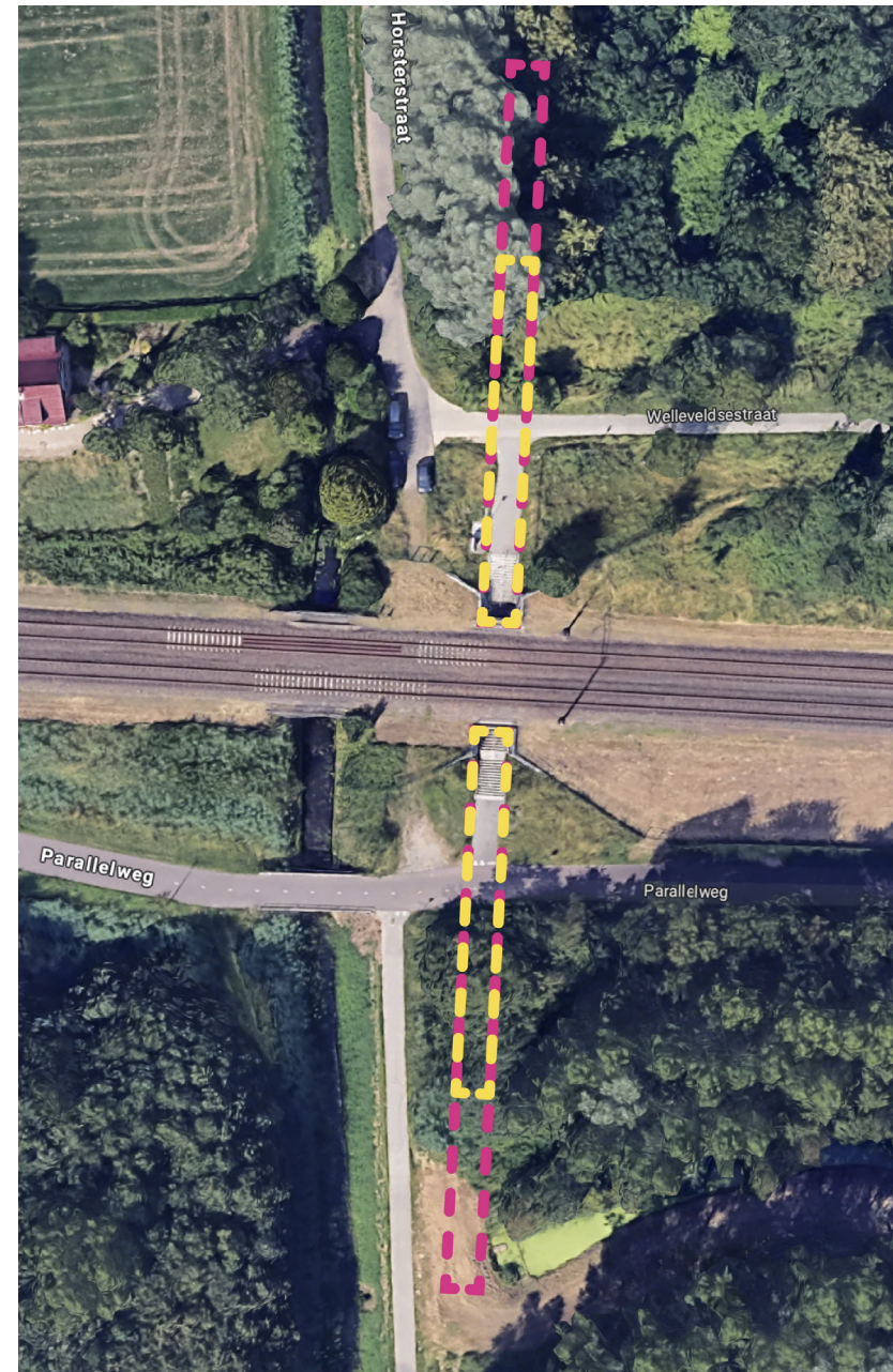
Voorbeelduitwerking met indicatie lengte mogelijke fietstunnel met een helling van 1:10 (geel) of 1:20 (roze).
