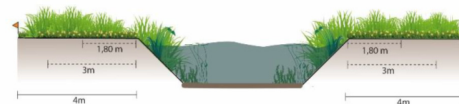
Doorsnedes natuurlijke onderhoudspaden (Waterschap Rijn & IJssel, Visie op onderhoudspaden)
